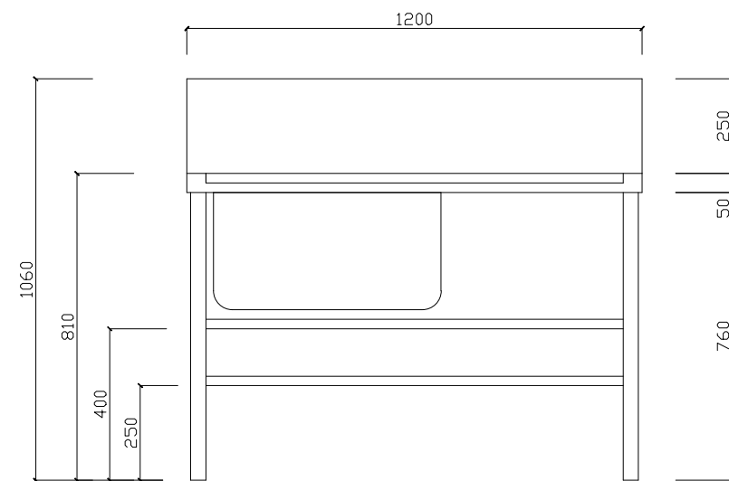
MẶT ĐỨNG
