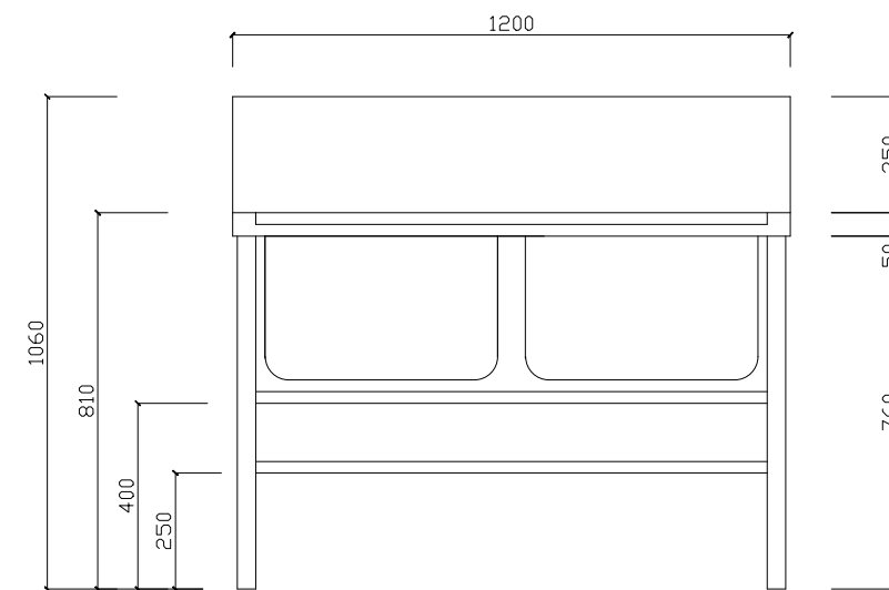
MẶT ĐỨNG
