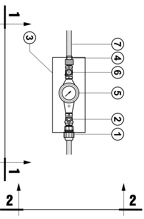
MẶT BẰNG ĐỘNG HỒ NƯỚC
