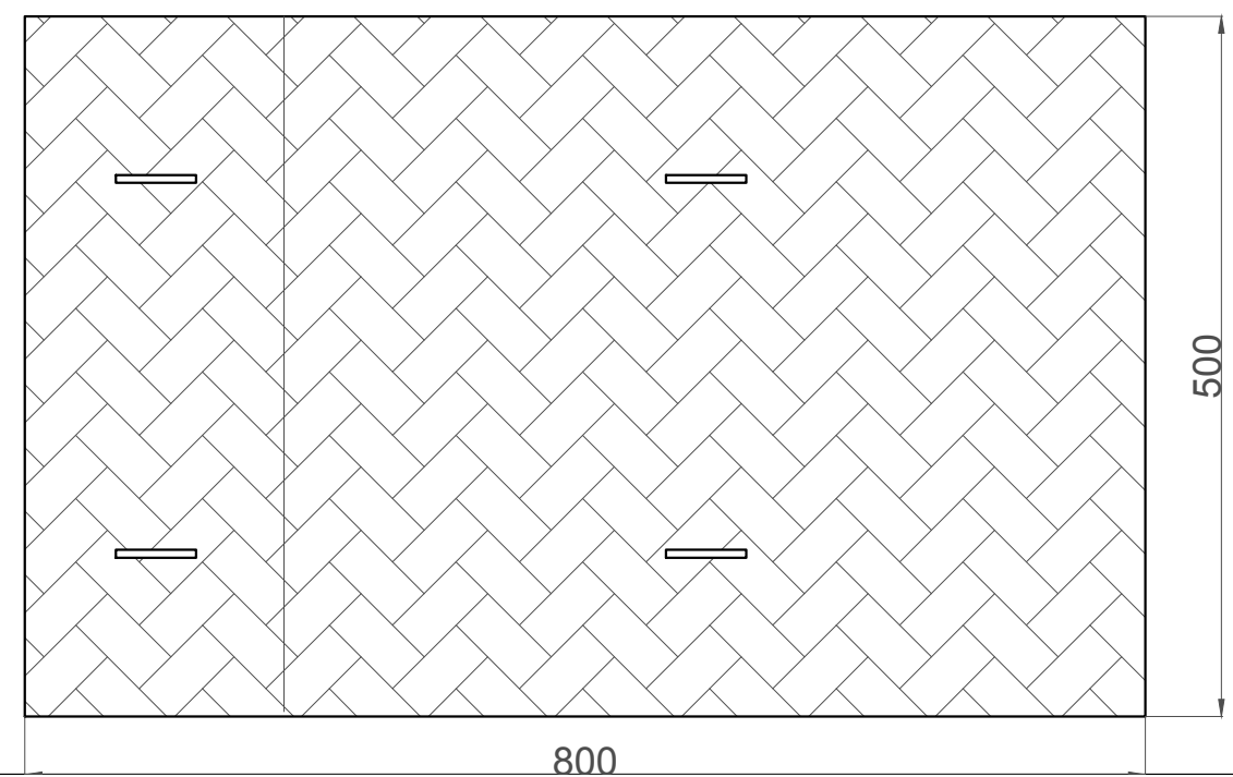
MẶT BẰNG NẮP
