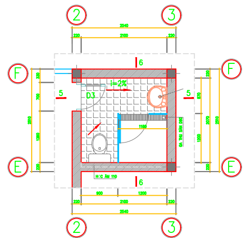
MẶT BẰNG WC3
