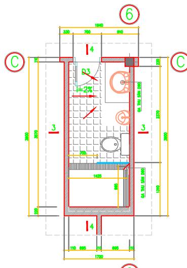
MẶT BẰNG WC2
