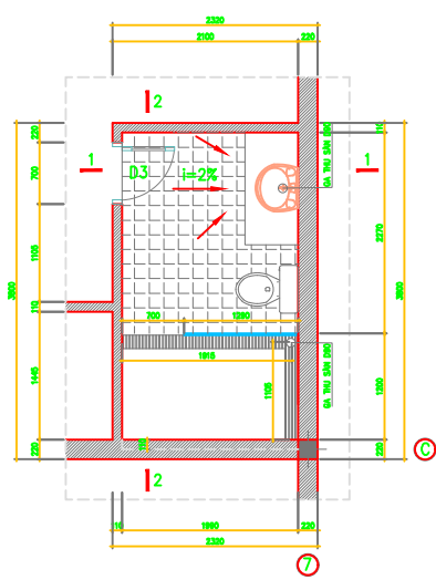
MẶT BẰNG WC1
