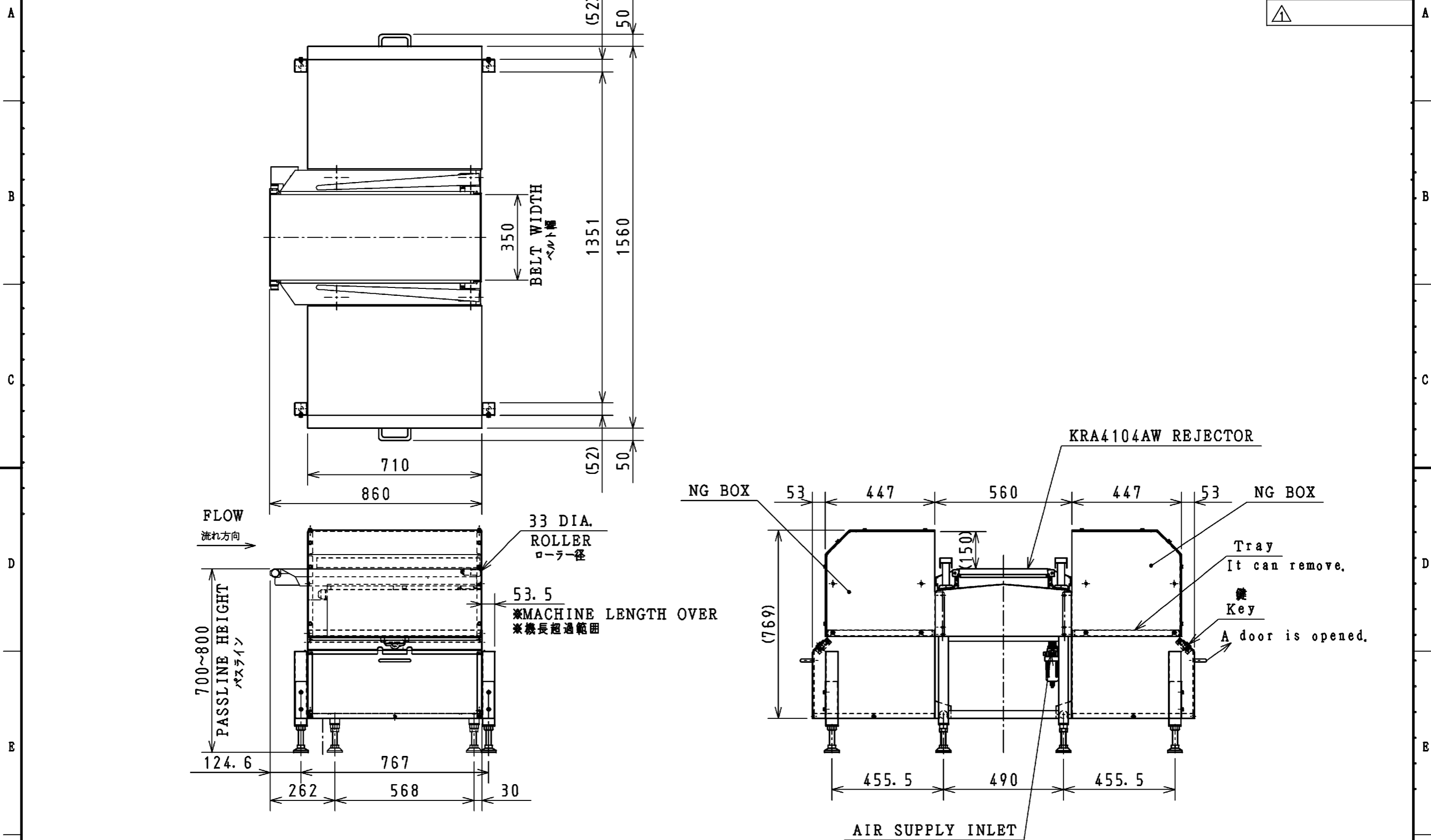
KRA4104AW REJECTOR (NGBOX WITH DOOR AND LOCK) KRA4104AW 選別機外観図 (扉付脚付NGボックス) (SCALE=1:15, 尺度=1:15)
