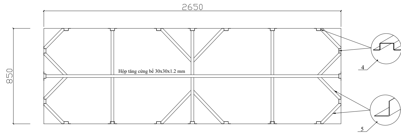
MẶT BẰNG KHUNG ĐỒ TRONG BỂ
