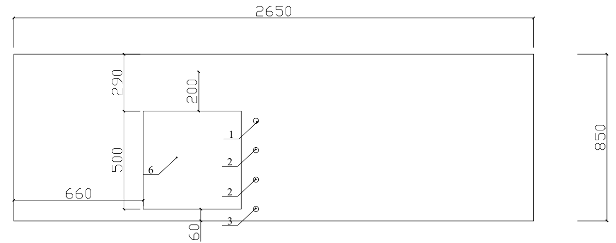
MẶT BẰNG NÁP BỂ
