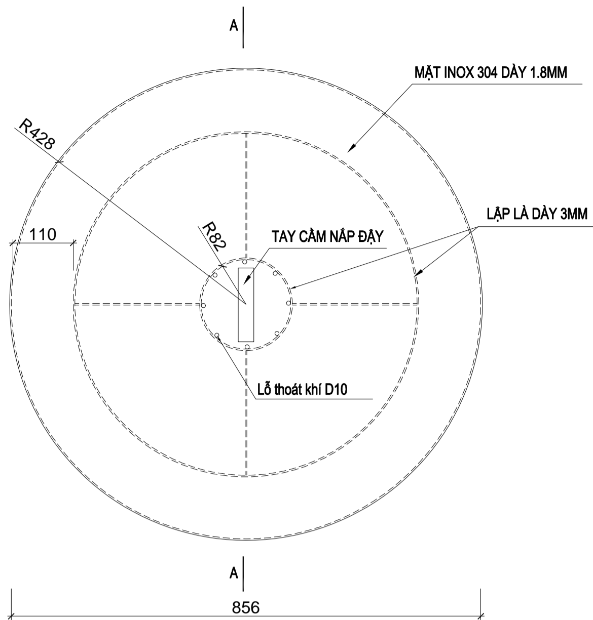
MẶT BẰNG NẮP GIẾNG
