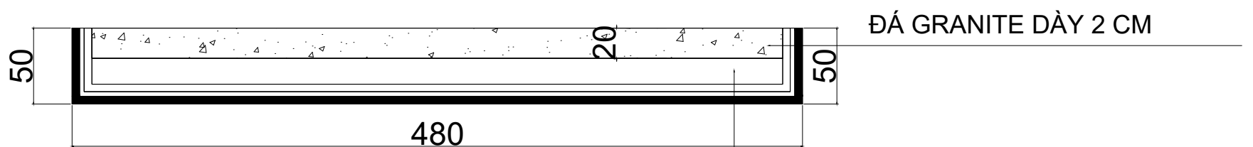
MẶT CẮT HỐ GA GẦN CÔNG
