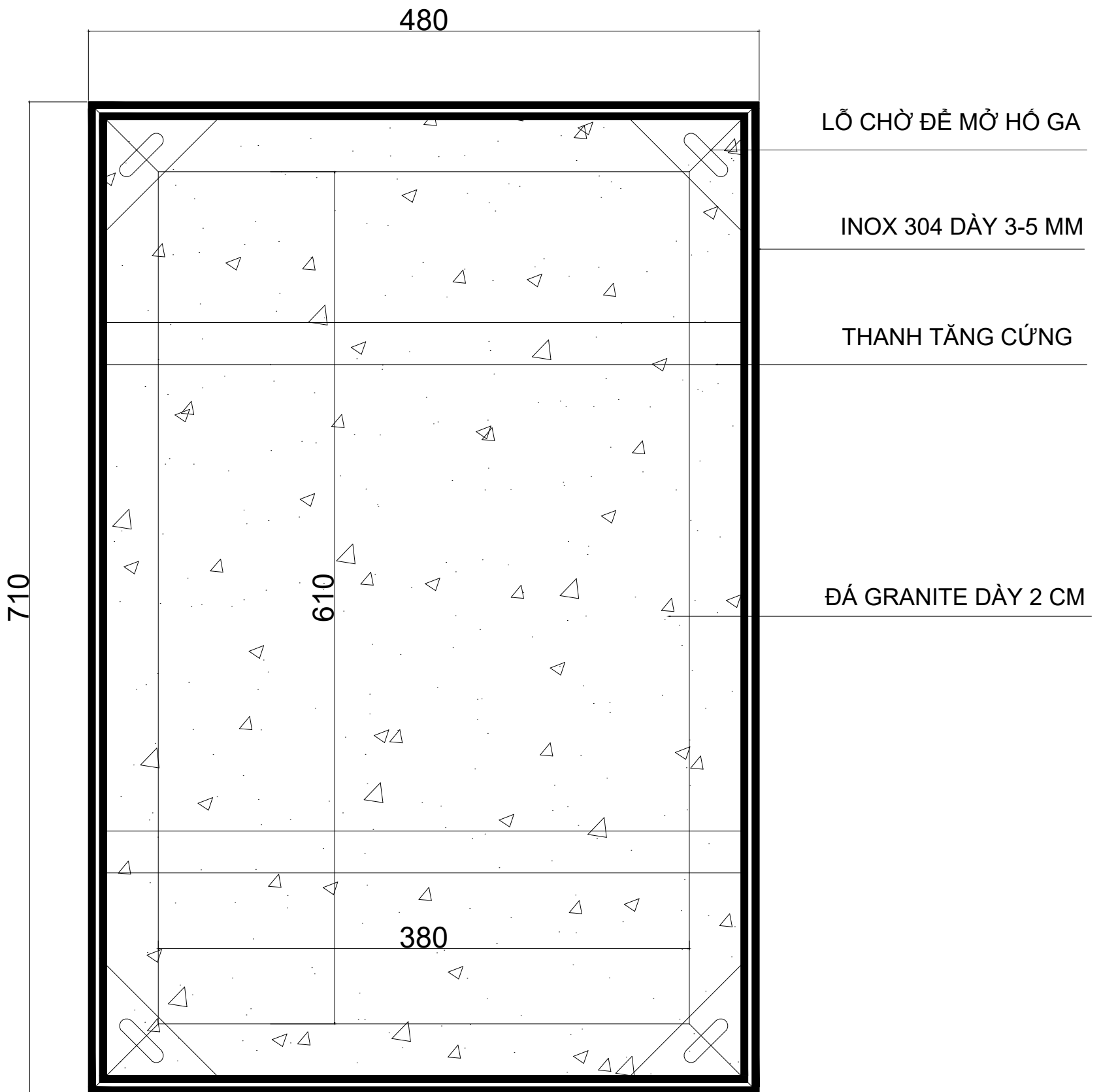
MẶT BẰNG HỐ GA GẦN CÔNG
