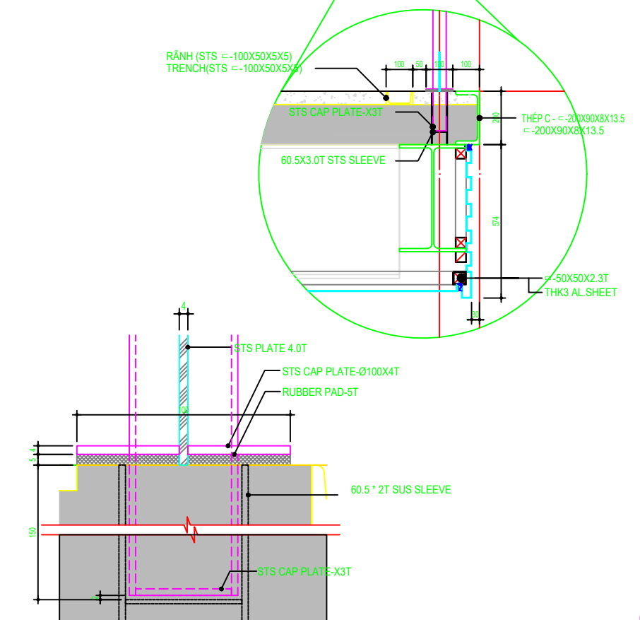
2 A - MẶT CẮT LỐI VÀO THIẾT BỊ 2 MỞ RỘNG TL 1/60 #2 EQUIP. ENTRANCE ENLARGED SECTION SC 1/60
