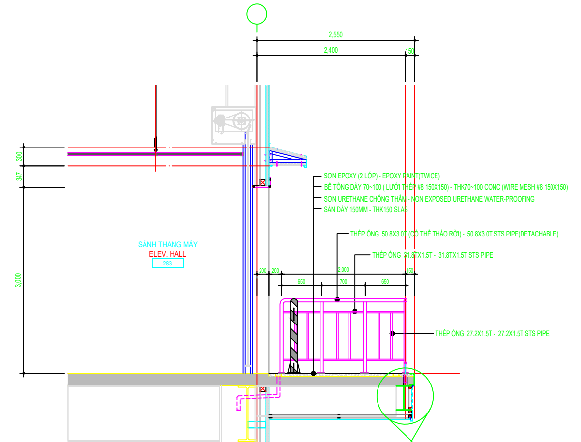
2 A - MẶT CẮT LỐI VÀO THIẾT BỊ 2 MỞ RỘNG TL 1/60 #2 EQUIP. ENTRANCE ENLARGED SECTION SC 1/60
