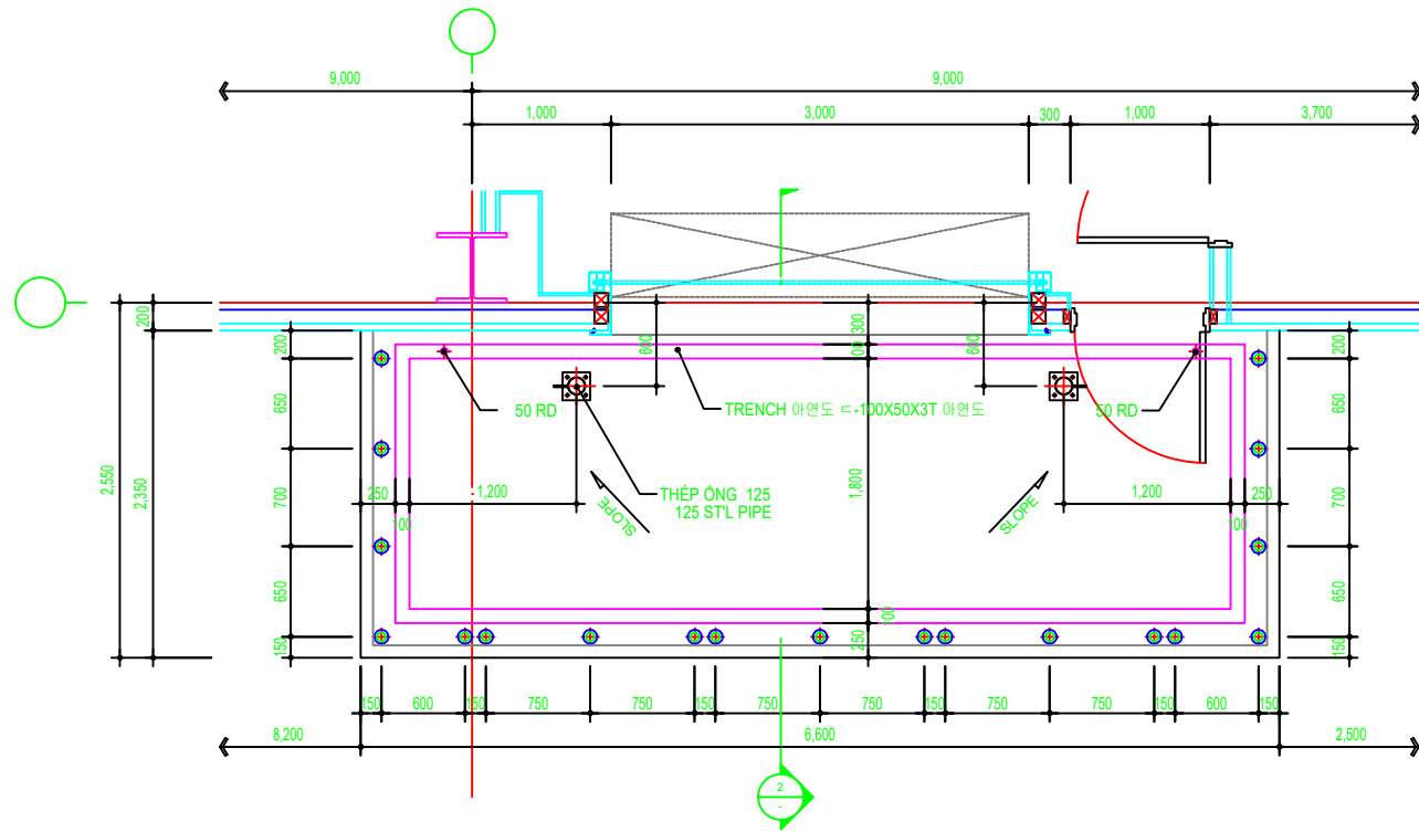
1 A - MẶT BẰNG LỐI VÀO THIẾT BỊ 2 MỞ RỘNG TL 1/60 #2 EQUIP. ENTRANCE ENLARGED PLAN SC 1/60
