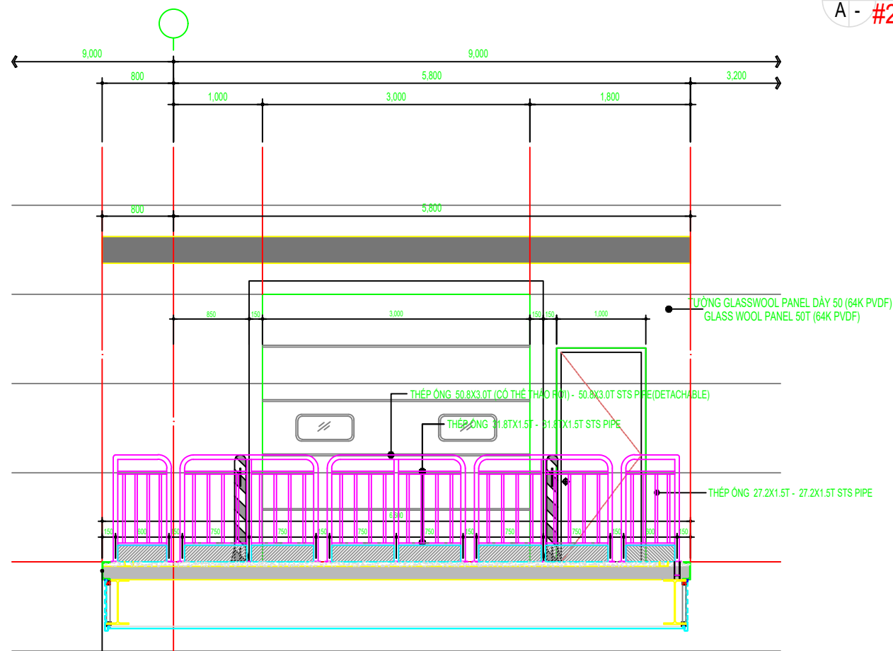
3 A - MẶT ĐỨNG LỐI VÀO THIẾT BỊ 2 MỞ RỘNG TL 1/60 #2 EQUIP. ENTRANCE ENLARGED ELEVATION SC 1/60
