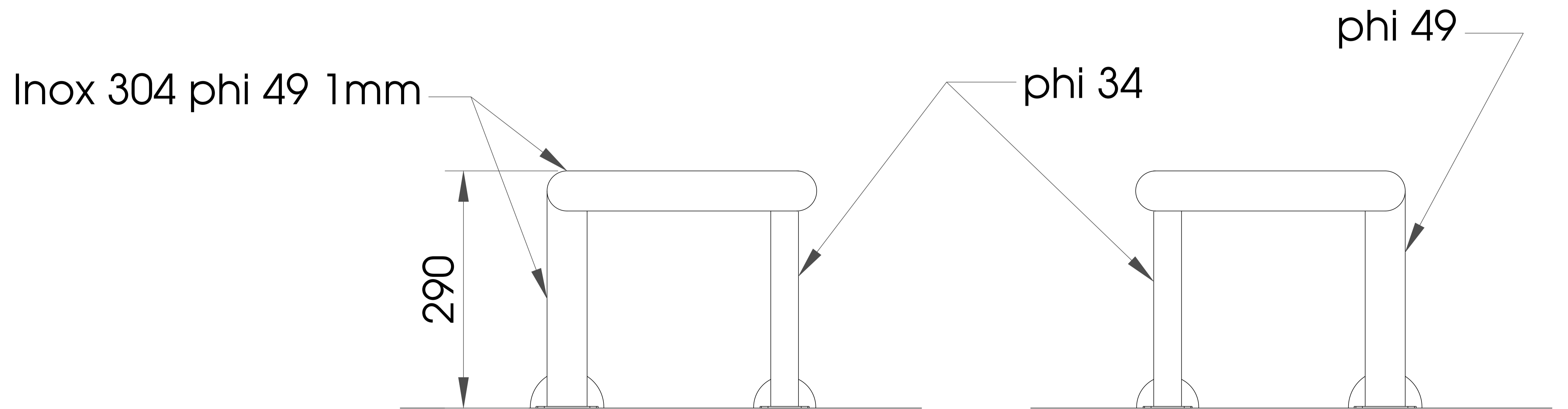
HÌNH CHIẾU CẠNH
