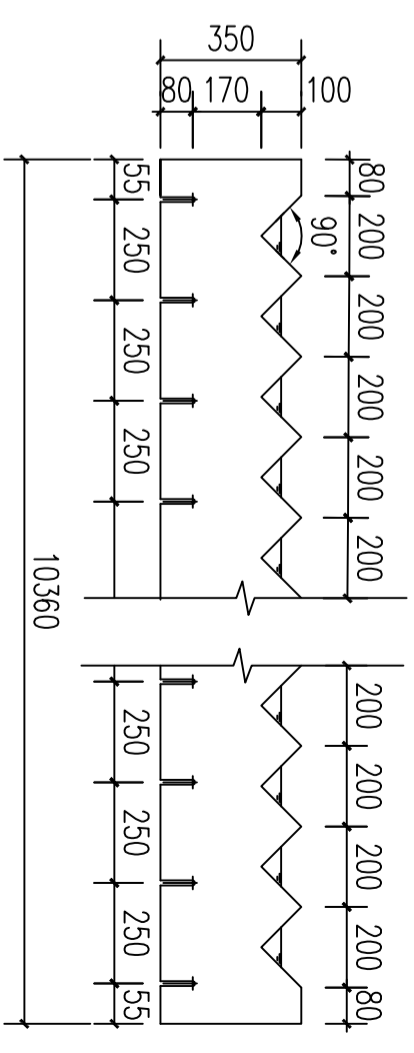
出水堰板 2:20
