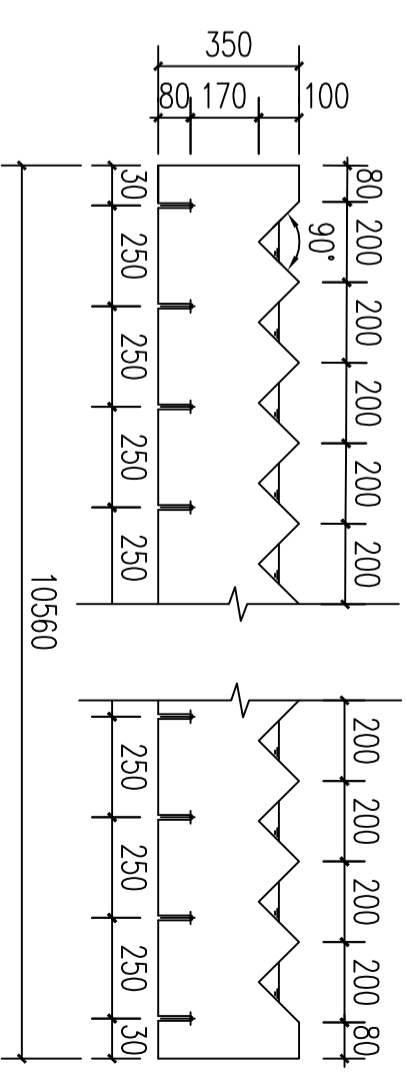
出水堰板 3:20
