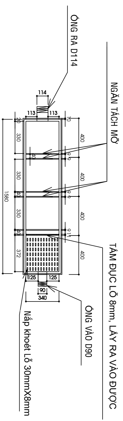
MẶT BẰNG BÊN TRONG HẦM TÁCH MỠ 4 NGĂN
