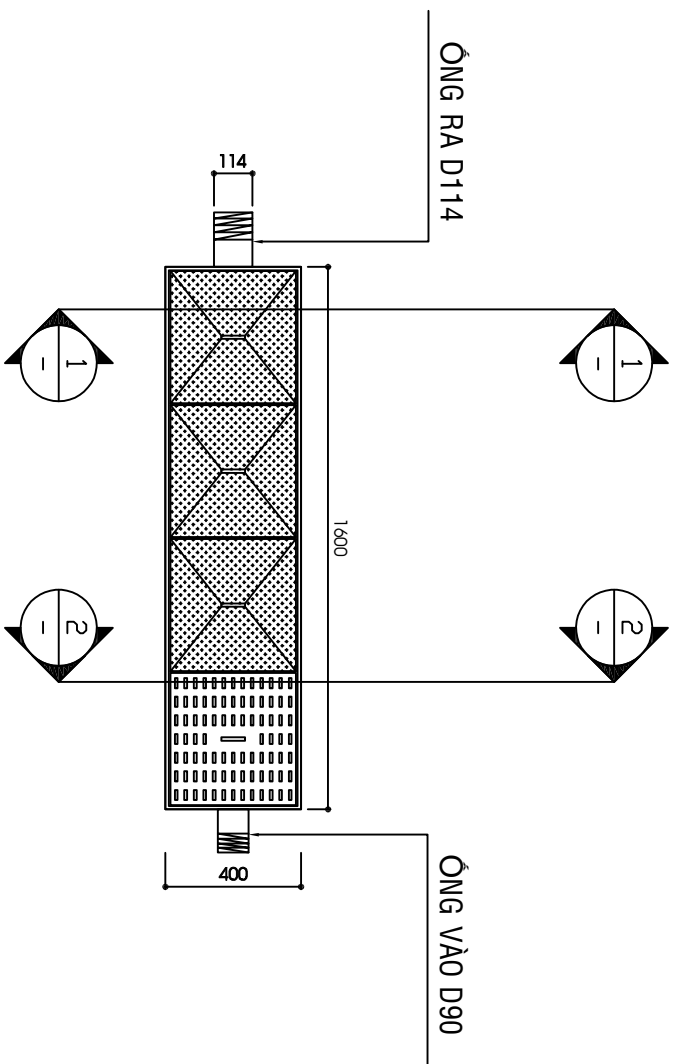
MẶT BẰNG NẬP HẦM TÁCH MỠ 4 NGĂN
