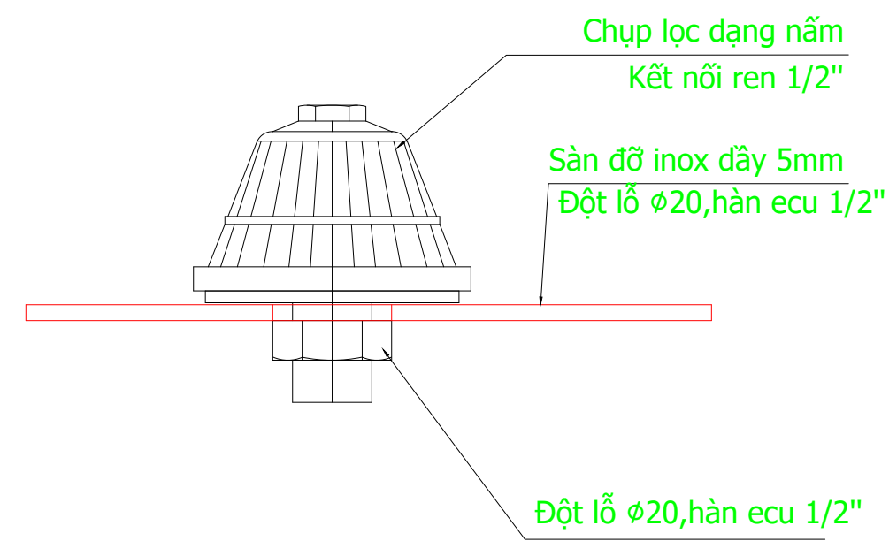
CHI TIẾT LỖ LẮP CHỤP LỌC
