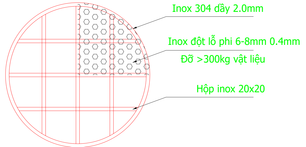
MẶT CẮT SÀN ĐỠ VẬT LIỆU
