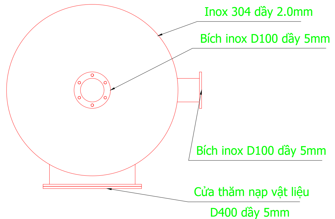
MẶT BẰNG THÁP KHÍ
