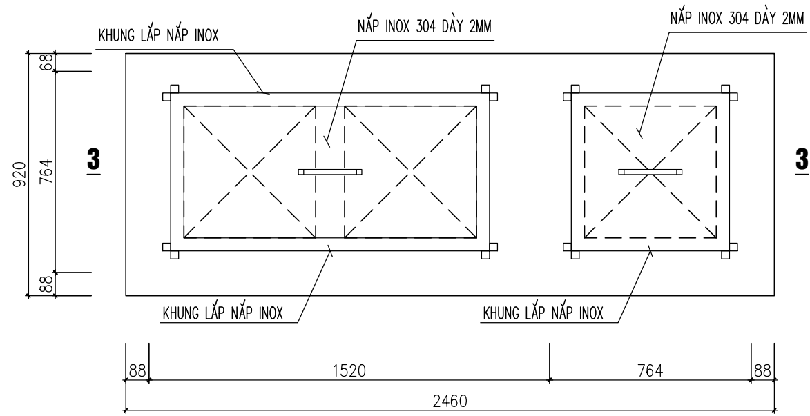
CHI TIẾT NẮP BỂ TÁCH MỠ
