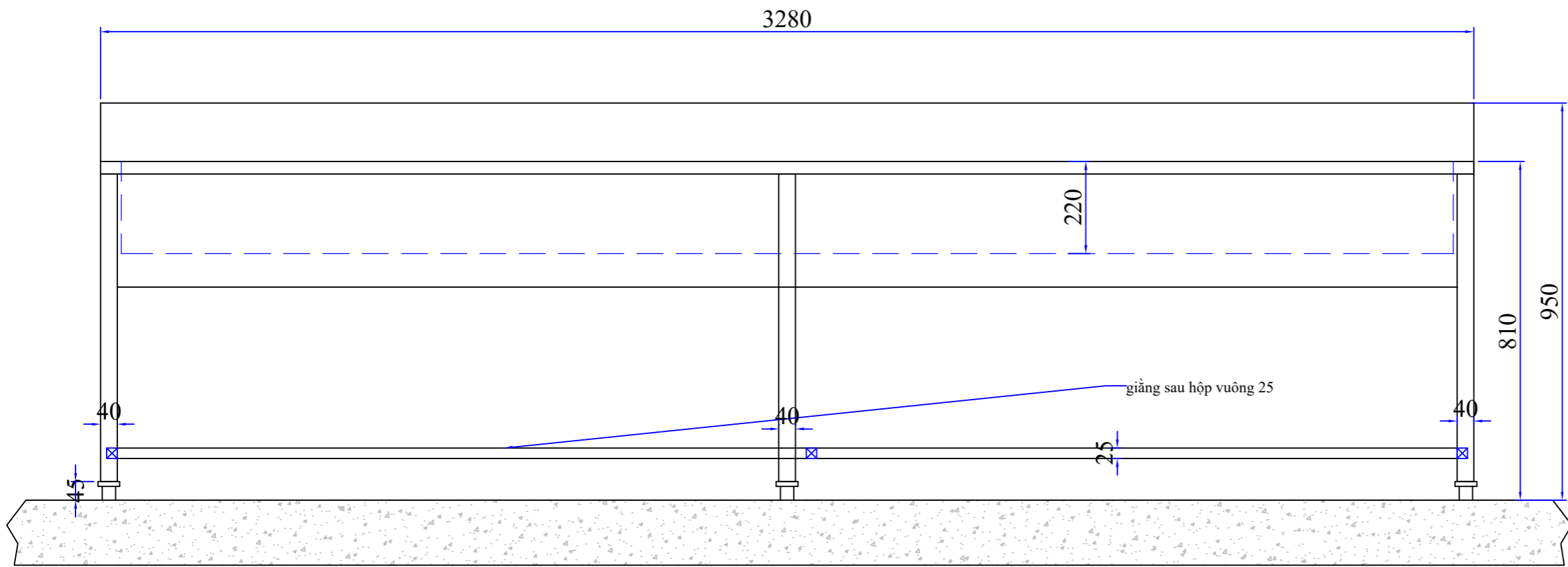
Mặt Đứng
