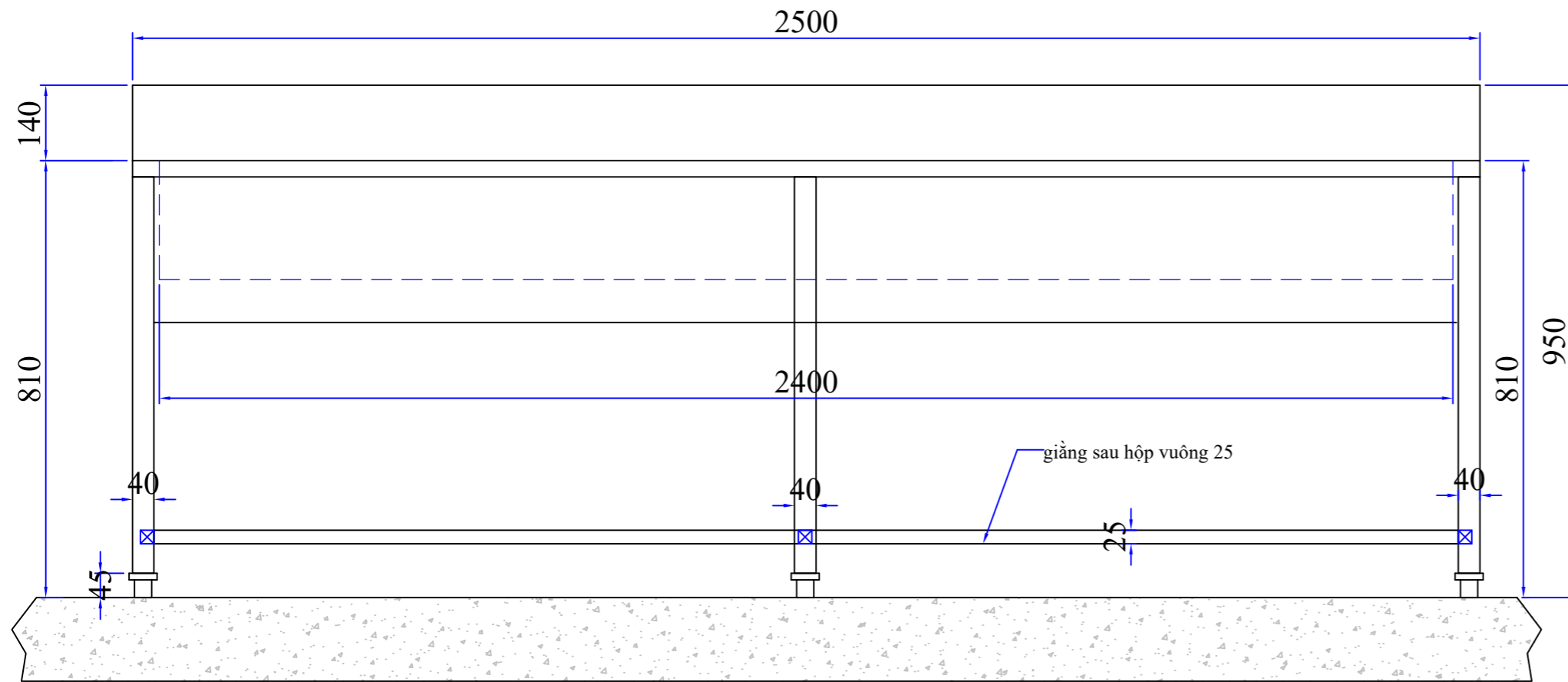
Mặt Đứng
