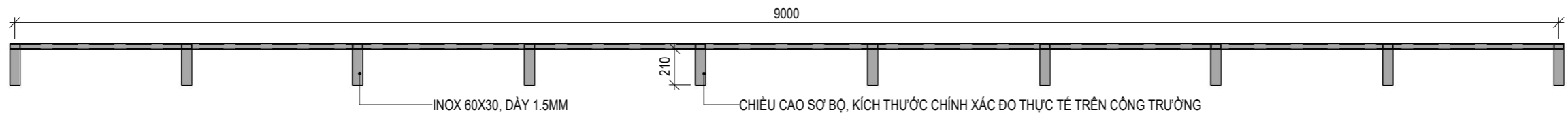
MẶT CẮT 1 GIÁ ĐỠ DÀN NÓNG ĐIỀU HÒA VÀ HEATPUMB
