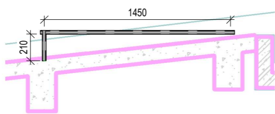
MẶT CẮT 2 GIÁ ĐỠ DÀN NÓNG ĐIỀU HÒA VÀ HEATPUMB
