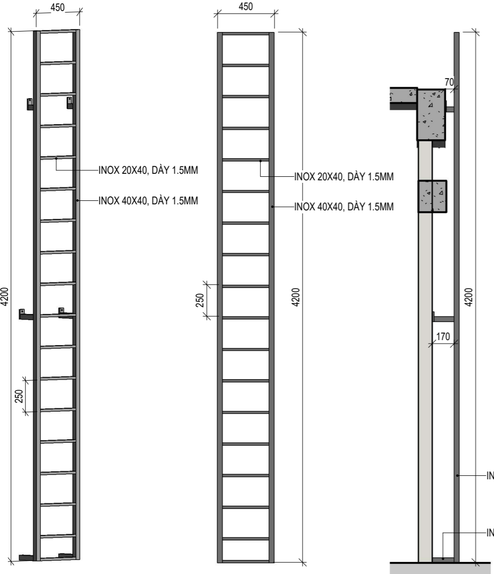
3D THANG LÊN MÁI
