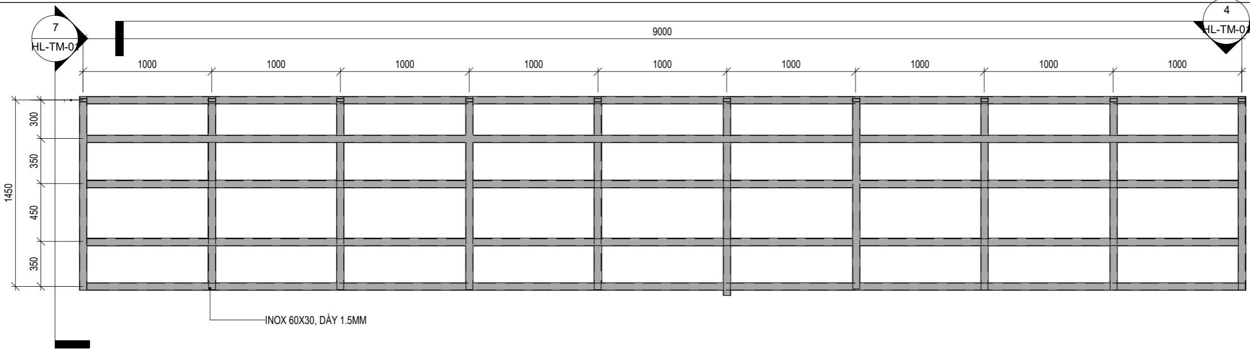
MẶT BẰNG GIÁ ĐỠ DÀN NÓNG ĐIỀU HÒA VÀ HEATPUMB
