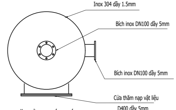
MẶT BẰNG THÁP KHÍ
