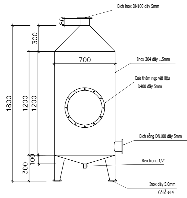
MẶT ĐÚNG THÁP KHÍ
