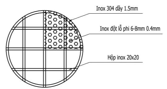
MẶT CẮT SÀN DỠ VẬT LIỆU
