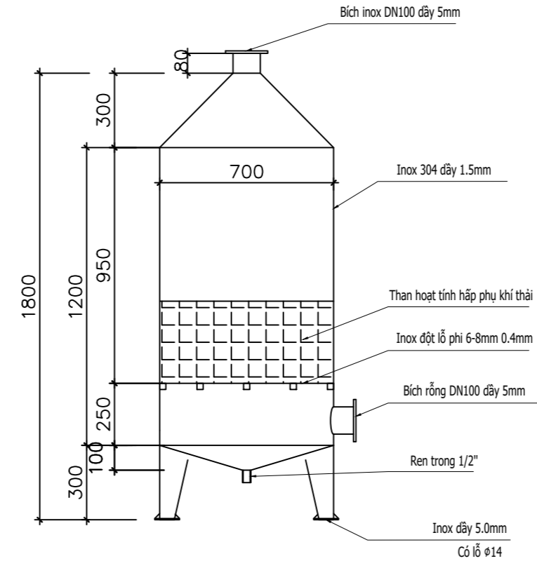
MẶT CẮT ĐÚNG THÁP KHÍ
